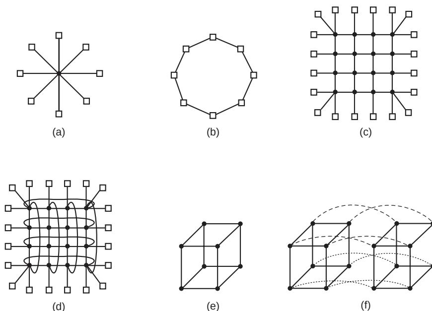
Figura 8-16. Varias topologías de interconexión. (a) Un solo switch. (b) Un anillo. (c) Una rejilla. (d) Un doble toroide. (e) Un cubo. (f) Un hipercubo 4D.
